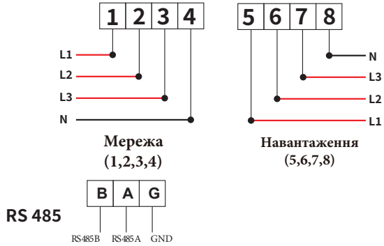
Рис. 7.20 Лічильник Eastron
