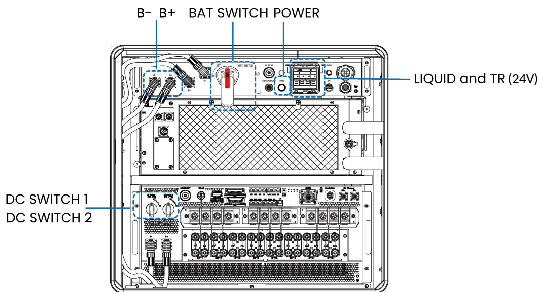
Внутрішня схема нижньої коробки корпусу
