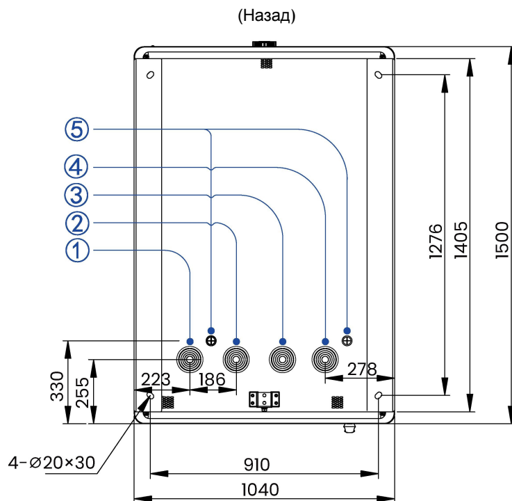
Монтажні отвори в нижній пластині (вид зверху) (одиниця виміру: мм)
